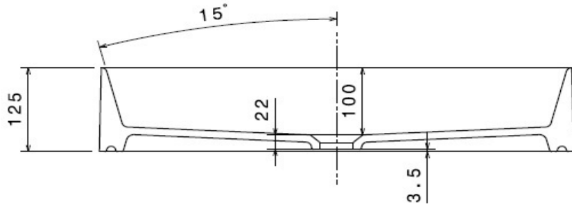
Sezione A-A Scala: 1:5
